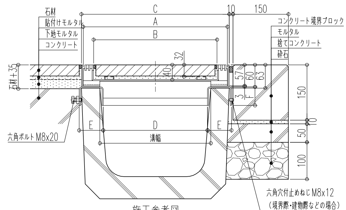
施工参考図
